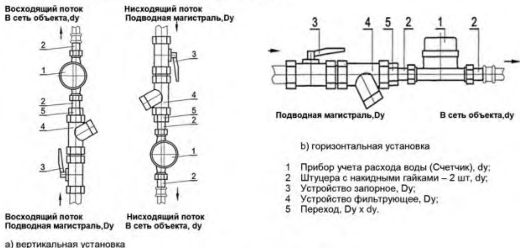
Рисунок 1 - Варианты подключения Счетчика
